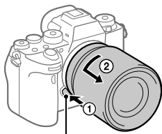
Objektiivin vapautuspainike
